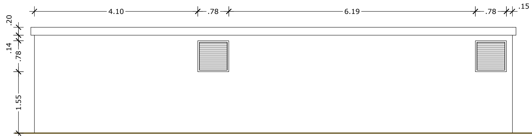
Arrière
