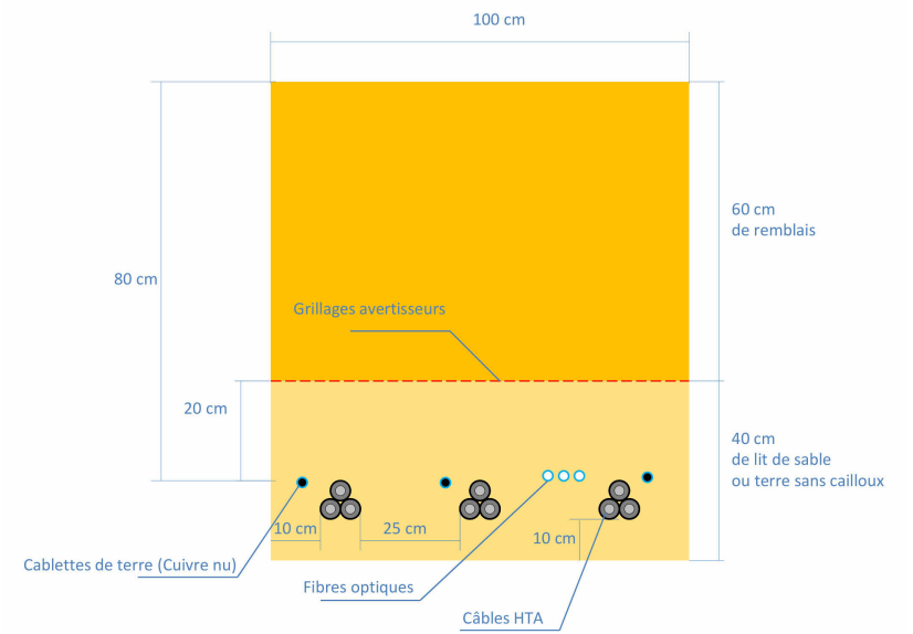
Coupe de principe d'enfouissement du câblage Échelle : 1/20
