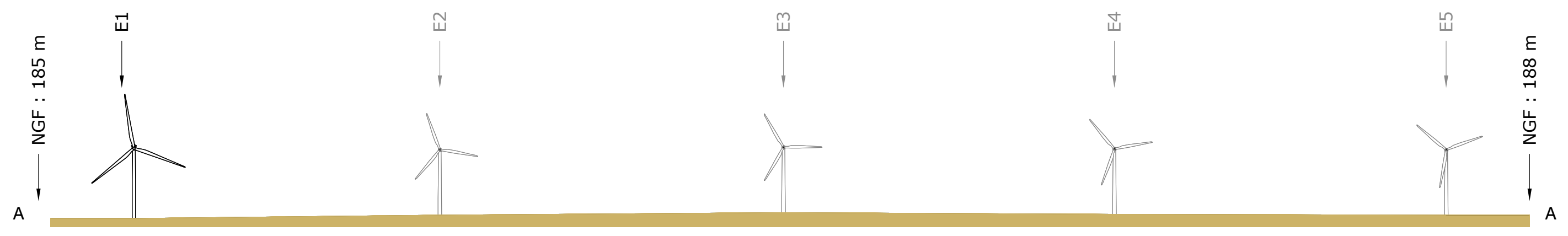
Coupe AA
